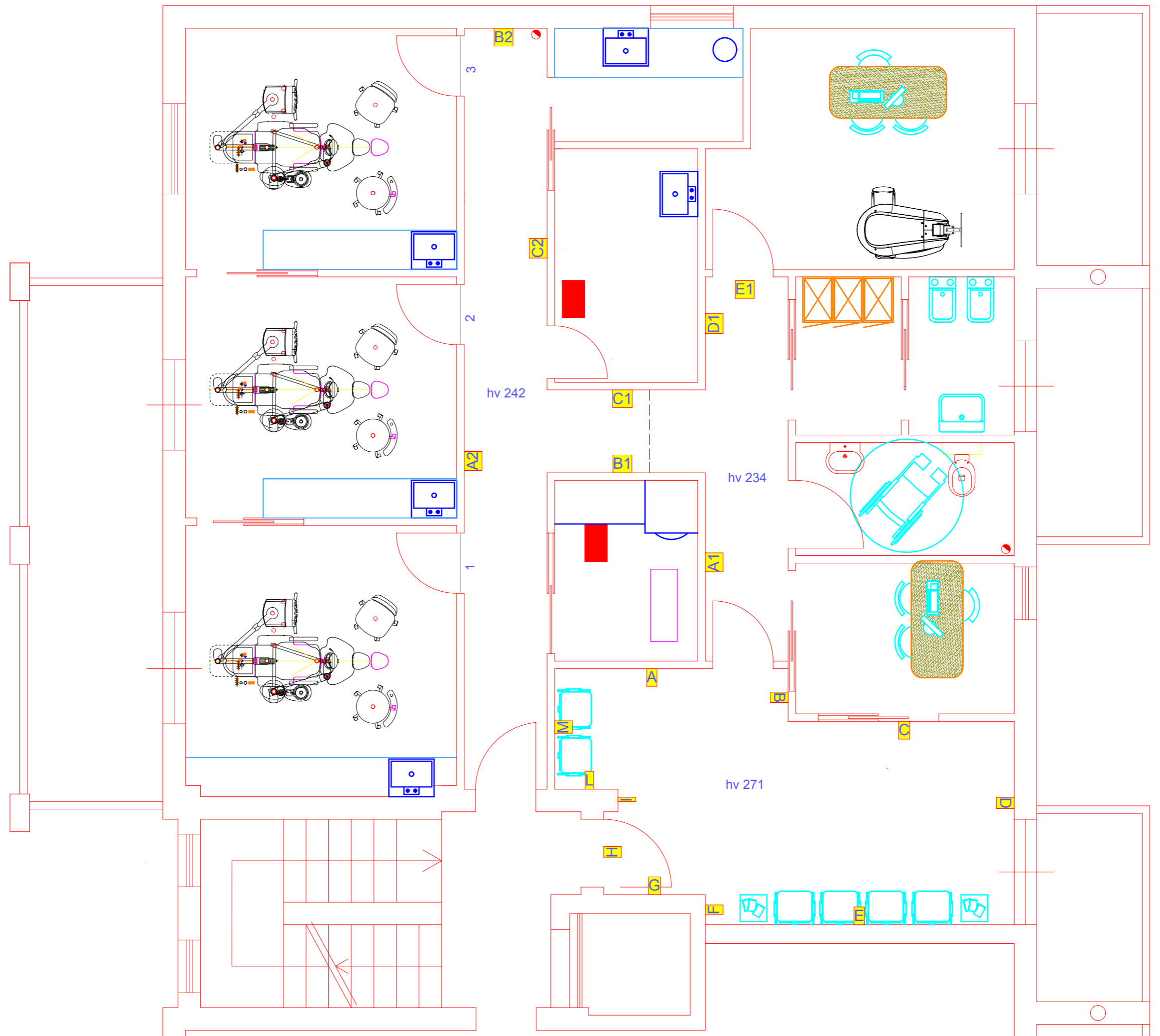
STUDIO DENTISTICO - PIANTE DELLE ATTREZZATURE 1/50
